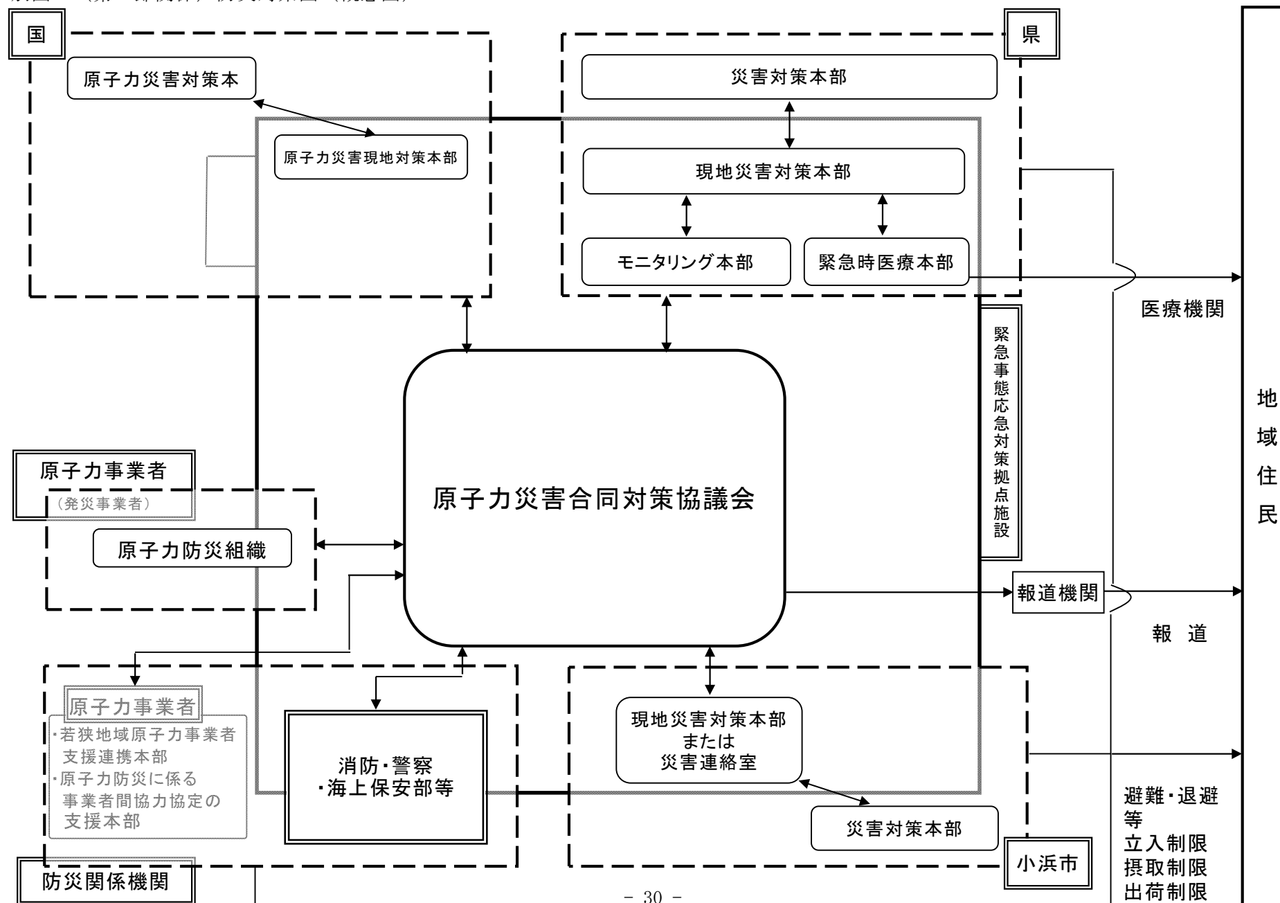
別図1（第3節関係）防災対策図（概念図）
