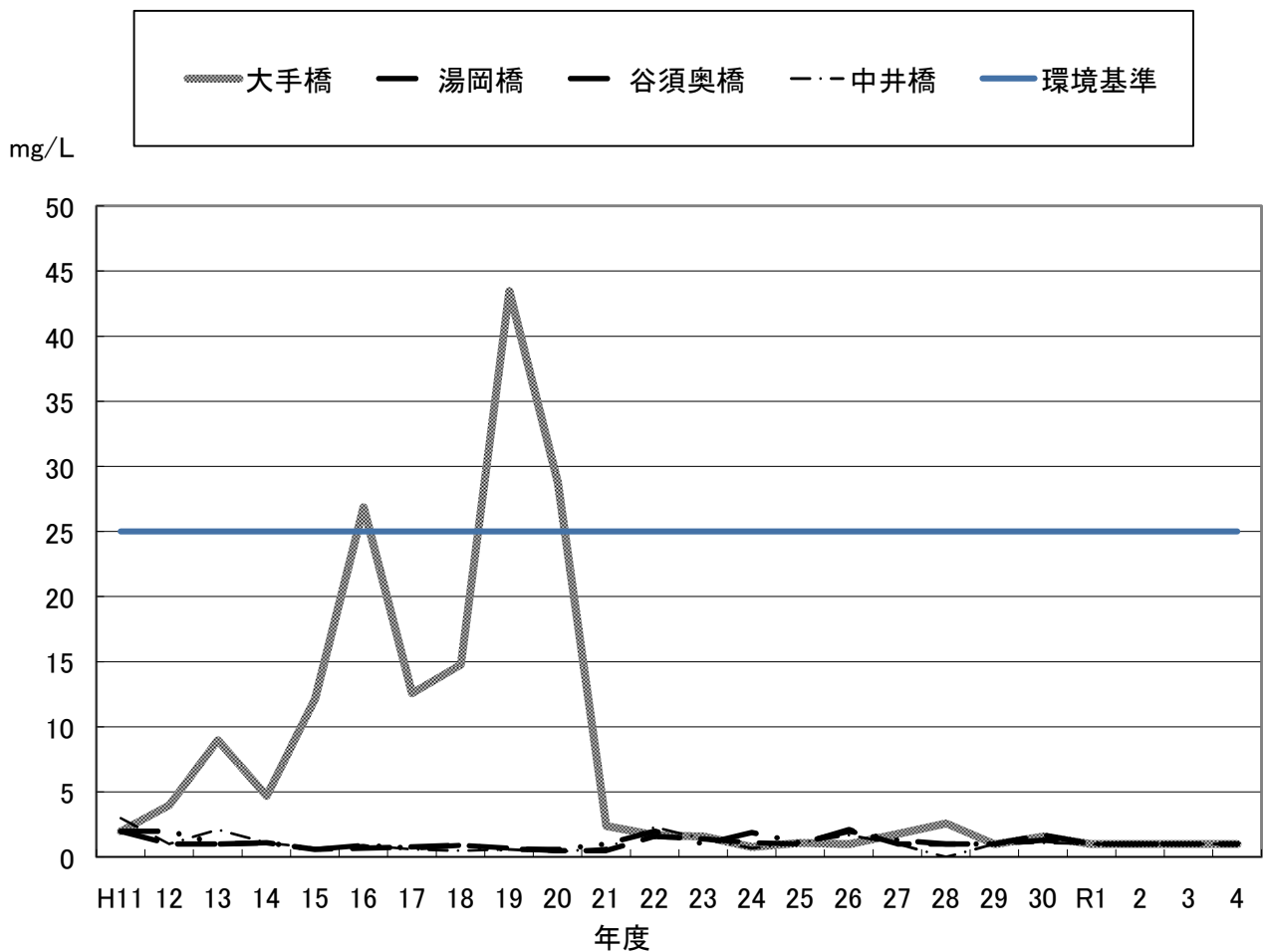
図. 5-7 南川各地点のSS経年変化
