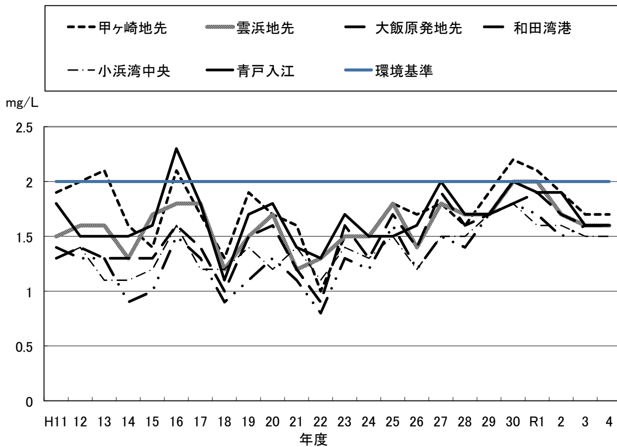
図. 5-8 小浜湾海域のCOD経年変化
