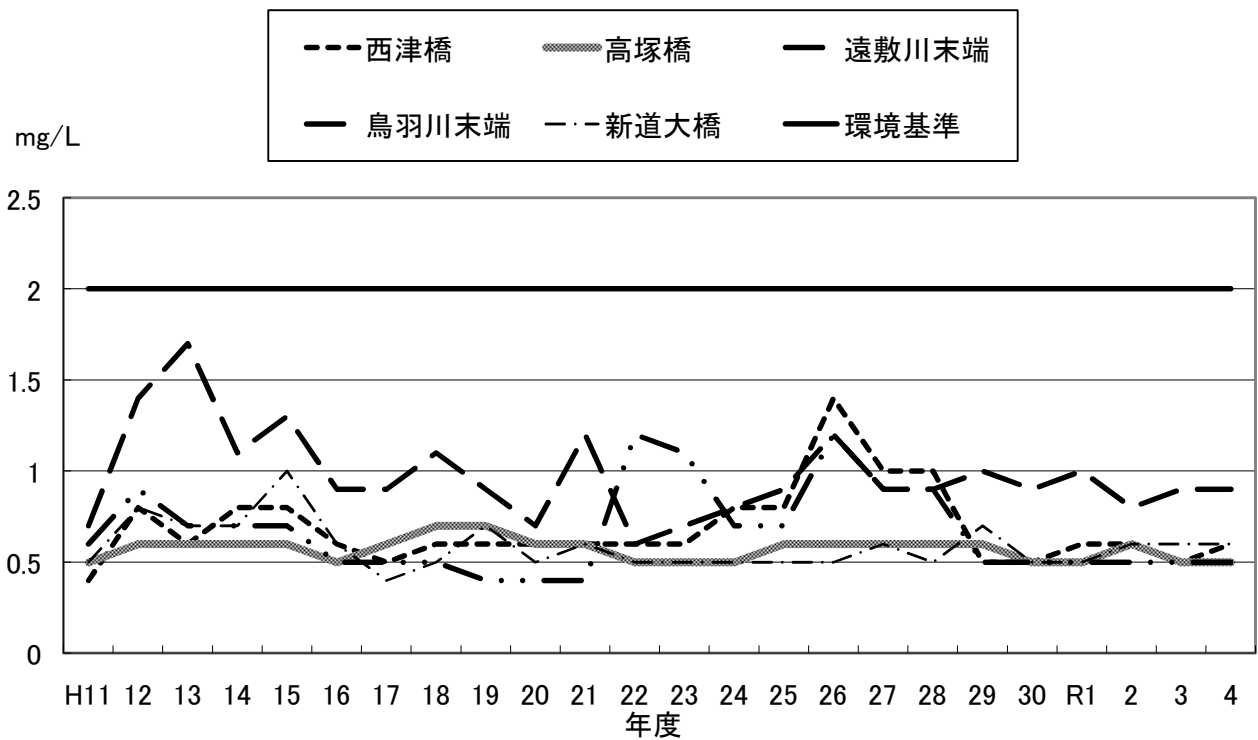
図. 5-4 北川各地点のBOD経年変化
