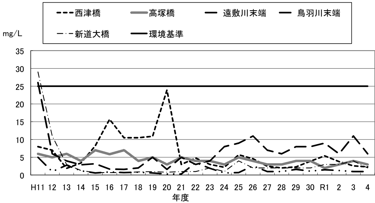
図. 5-6 北川各地点のSS経年変化
