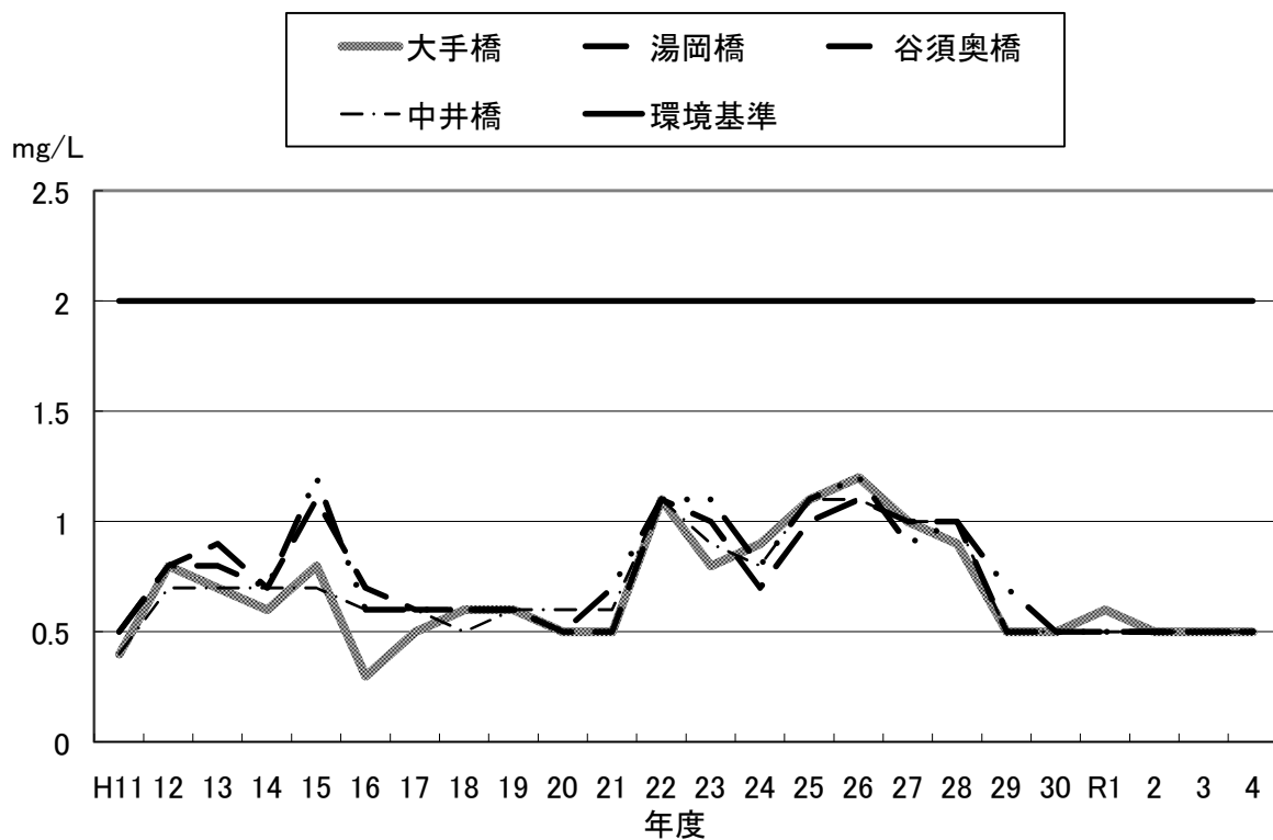
図. 5-5 南川各地点のBOD経年変化
